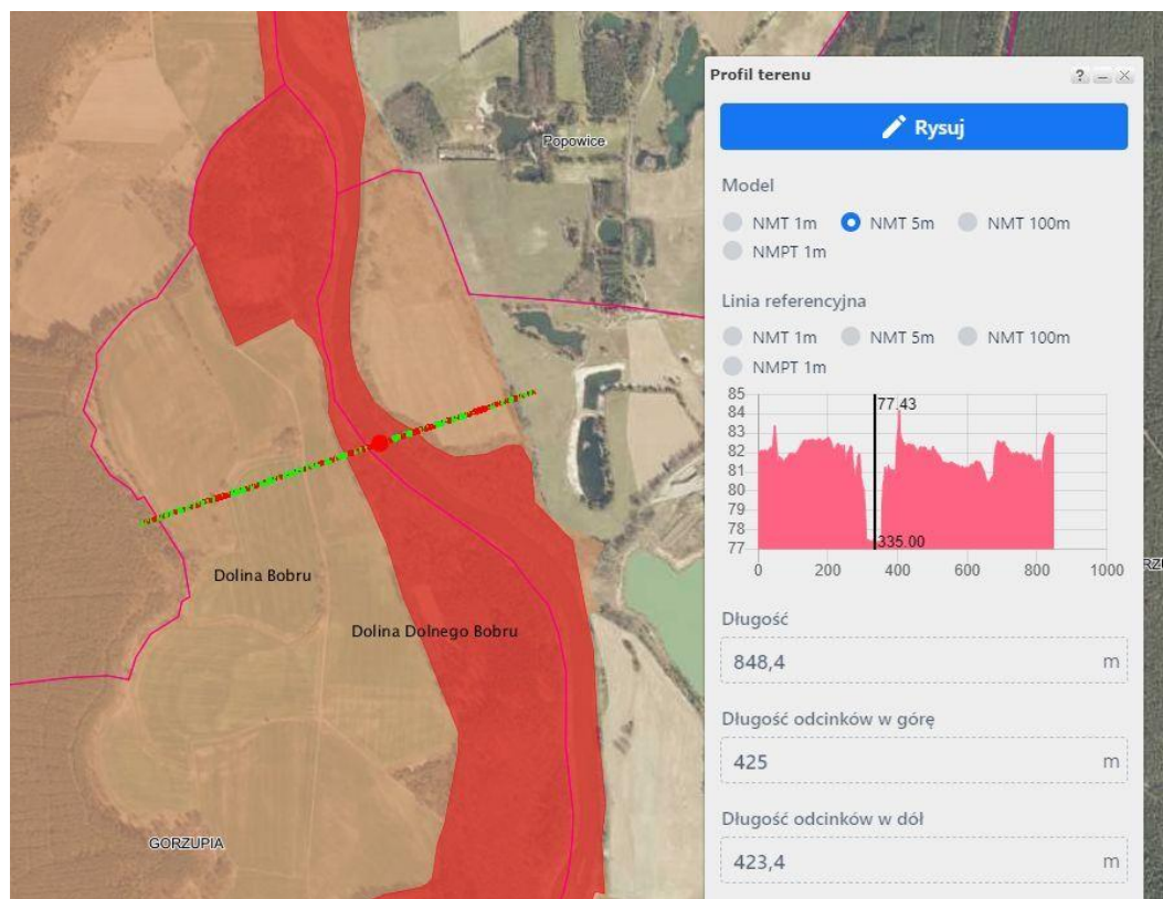
Profil terenu w Obszarze Chronionego Krajobrazu z zaznaczeniem rzędnej rzeki Bóbr w oparciu o dane geoportal.gov.pl
